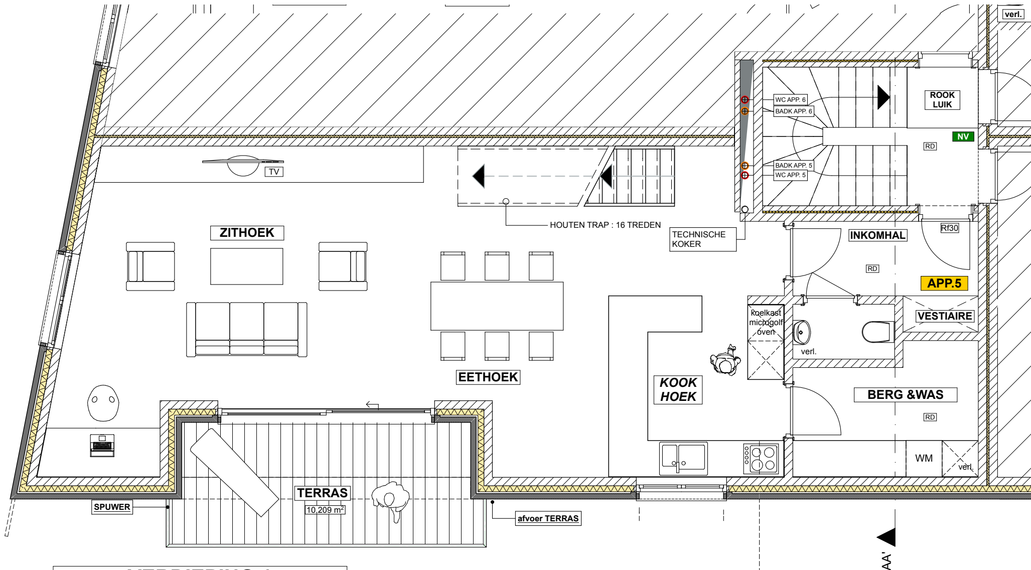
VERDIEPING 1 APPARTEMENT 5
